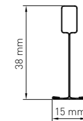
Hoofdprofiel
