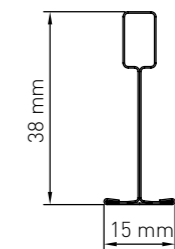
Tussenprofiel
